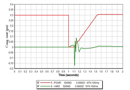
Hình 11. Công suất phát trong mô phỏng 1 (pu)
