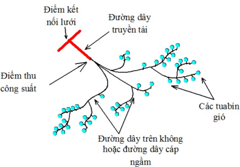
Hình 7. Mô hình đơn giản của một nhà máy điện gió kết nối lưới điện
