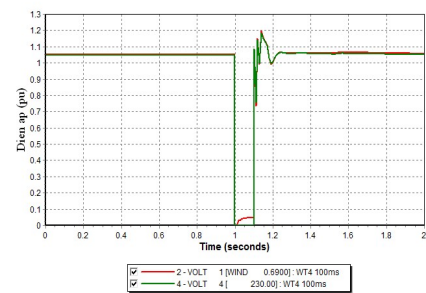
Hình 10. Điện áp trong mô phỏng 1 (pu)
