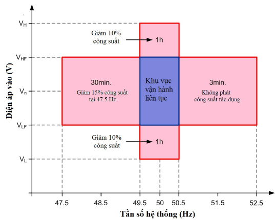
Hình 5. Điện áp - tần số làm việc của MPĐ gió
