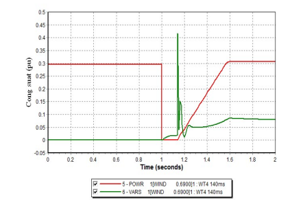
Hình 14. Công suất phát trong mô phỏng 2 (pu)
