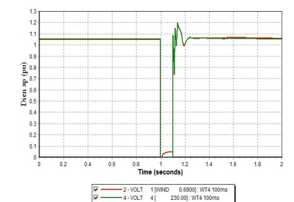
Hình 12. Điện áp trong mô phỏng 2 (pu)
