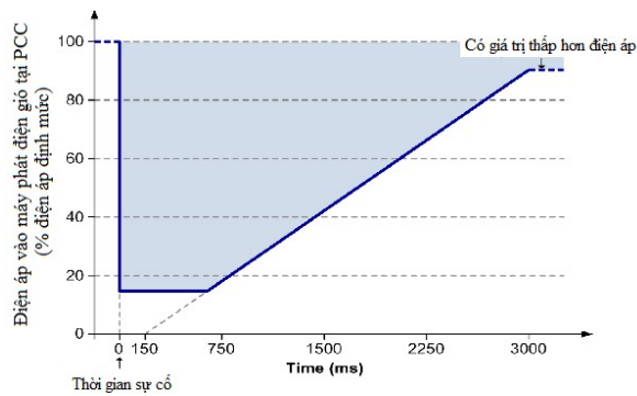
Hình 4. Khả năng phục hồi sau sự cố của một tuabin gió
