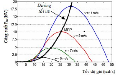
Hình 3. Đường đặc tính công suất - tốc độ gió của tuabin gió
