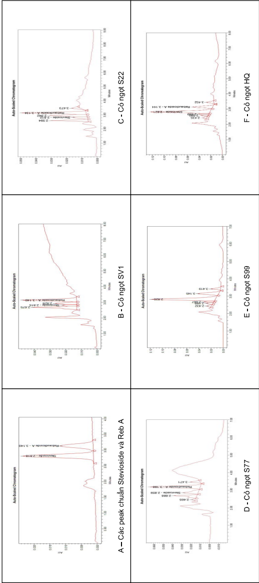
Hình 1. Sắc ký đồ của các chất chuẩn Stevioside và Reba (A); của các STG cỏ ngọt Việt Nam SV1 (B), S22 (C), S77 (D), S99 (E) và HQ của Hàn Quốc (F)
